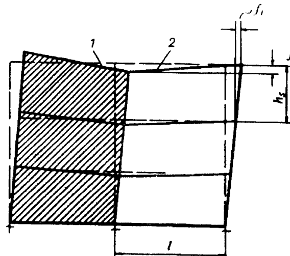
Черт. 6. Схема перекося этажных ячеек 2, примыкающих к диафрагмам жесткости l в зданиях со связевым каркасом (пунктиром показана исходная схема каркаса до приложения нагрузки)
