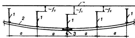
Черт. 5. Схема для определения прогибов стропильных конструкций при наличии подвесных крановых путей
