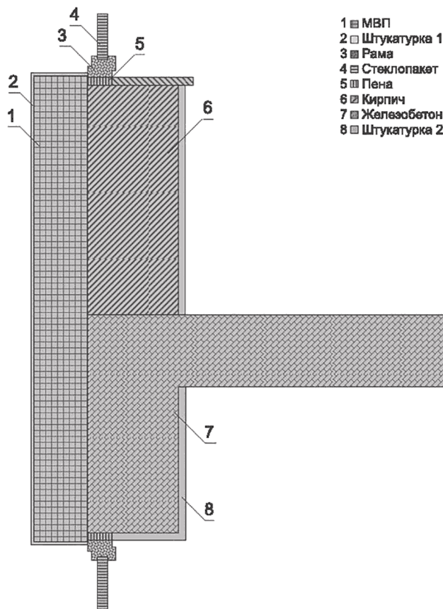
Рисунок И.1 — Схематическое изображение вертикального разреза стены с теплоизоляционным фасадом в зоне расположения светопроемов с оконными блоками
