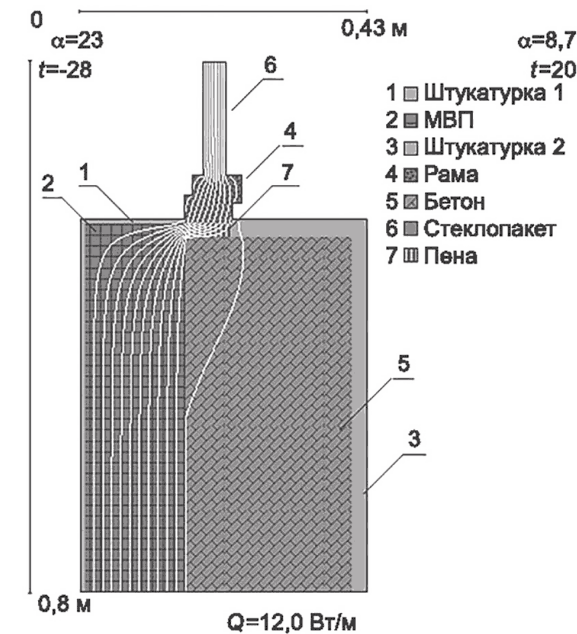
Рисунок И.2 — Температурное поле узла конструкции, содержащего линейный элемент 1
